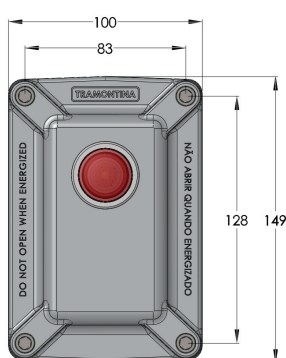
Vista superior
