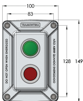
Vista superior
