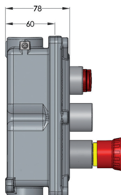
Vista lateral
