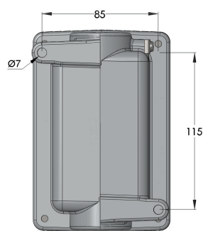
Vista inferior
