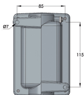
Vista inferior
